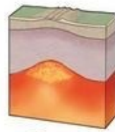
Ⓓ = Rift
